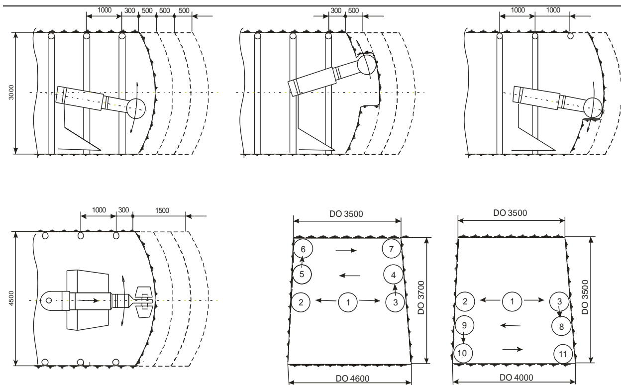
Slika 1. Izrada profila jamske prostorije sa mašinom AM 50 z-w po fazama
