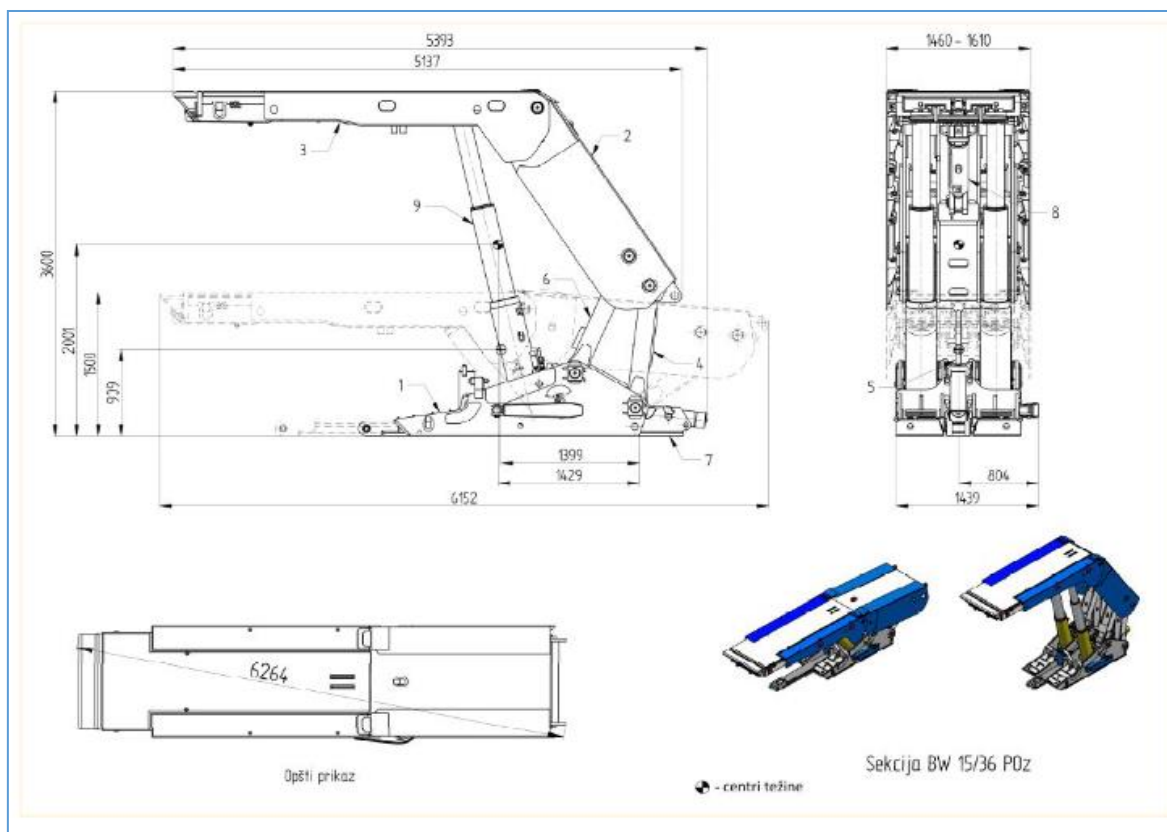
Slika 1. Sekcija BW 15/36 POz
